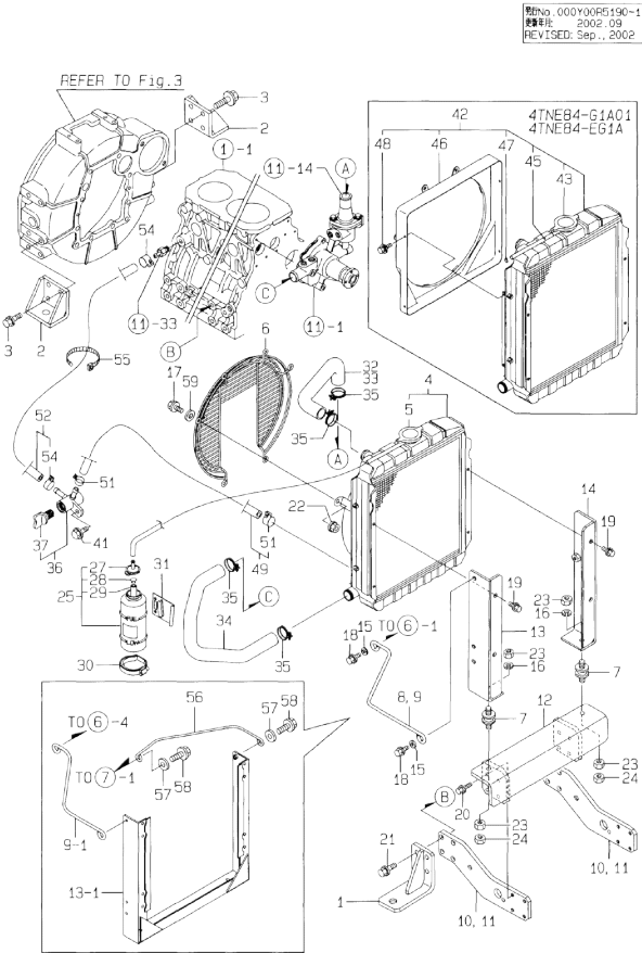
Fig.12. RADIATOR
